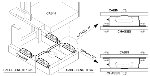
Montaj Detayları
