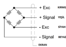
Kablo Bağlantısı
